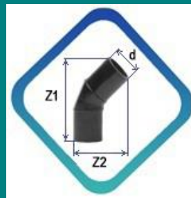
ОТВОД 45-60° ОДНОСЕКЦИОННЫЙ ПЭ 100 SDR 17 (PN 10)
