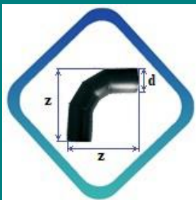
ОТВОД 90° ДВУХСЕКЦИОННЫЙ ПЭ 100 SDR 17 (PN 10)
